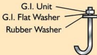
G.I. Hook Bolt
